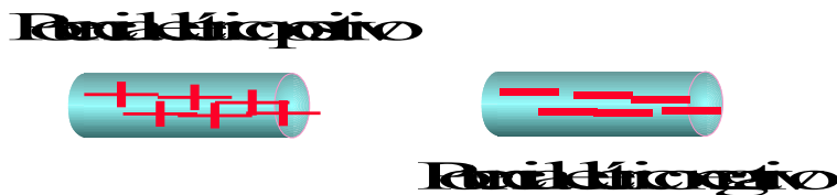
Fig.9 Corpos com potenciais elétricos positivos e negativos.
