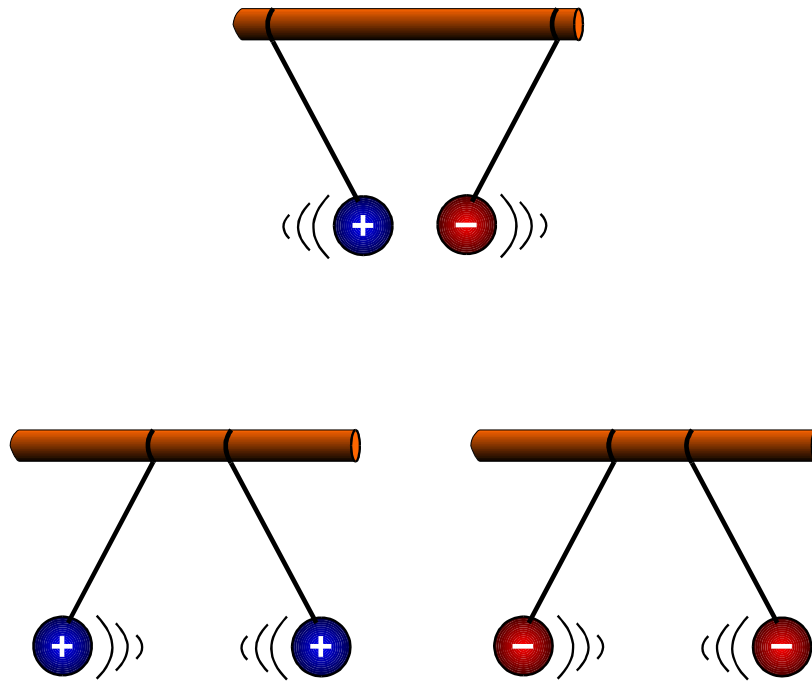
Fig.6 Interação entre corpos eletrizados.
