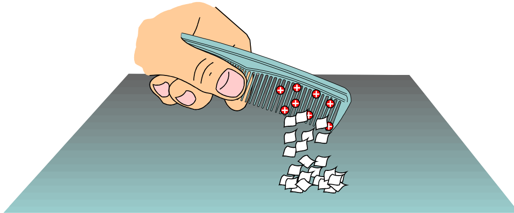
Fig.13 Pente fracamente atritado atrai menos papel.
