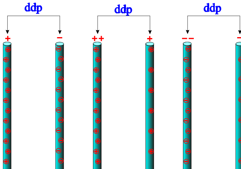
Fig.16 Diferença de potencial entre corpos eletrizados.
