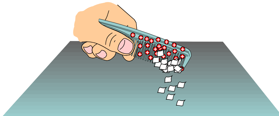
Fig.12 Pente fortemente atritado atrai mais papel.
