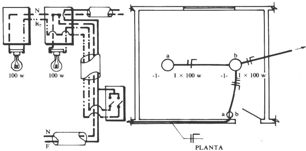
Dois lâmpadas acesas por um interruptor de duas seções, pelo qual chega a alimentação.
