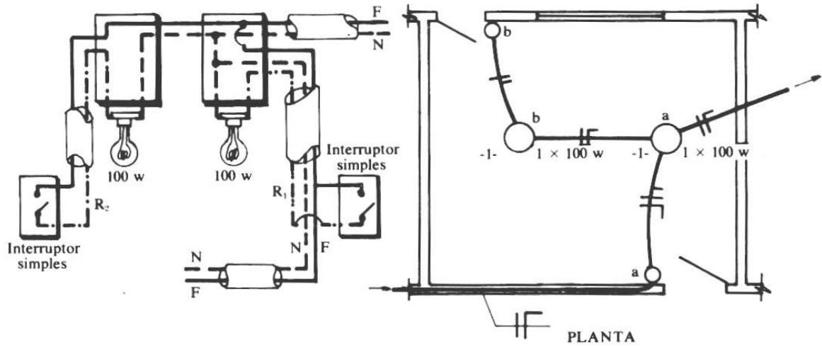
Duas lâmpadas comandadas por interruptores independentes, de uma seção cada.
