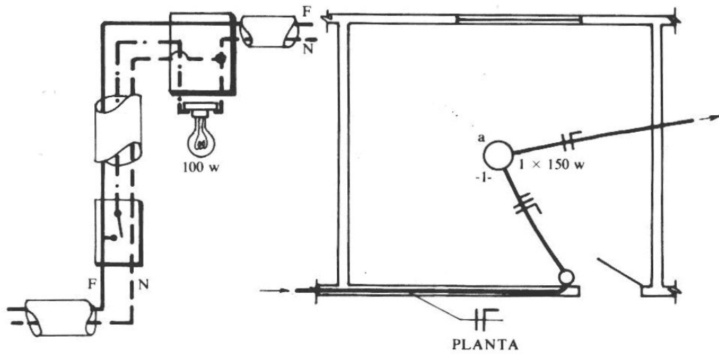
Lâmpada comandada por interruptor de uma seção, pelo qual chega alimentação.
