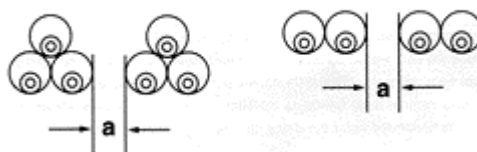
CABOS UNIPOLARES
