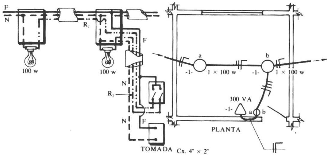
Dois pontos de luz comandados por um interruptor de duas seções e tomada.
