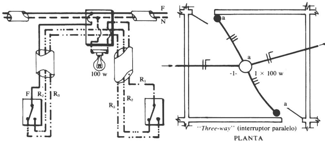
Lâmpada comandada por three-way
